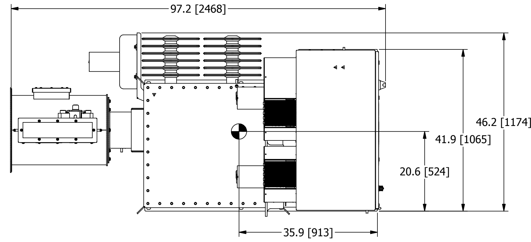
TOP
